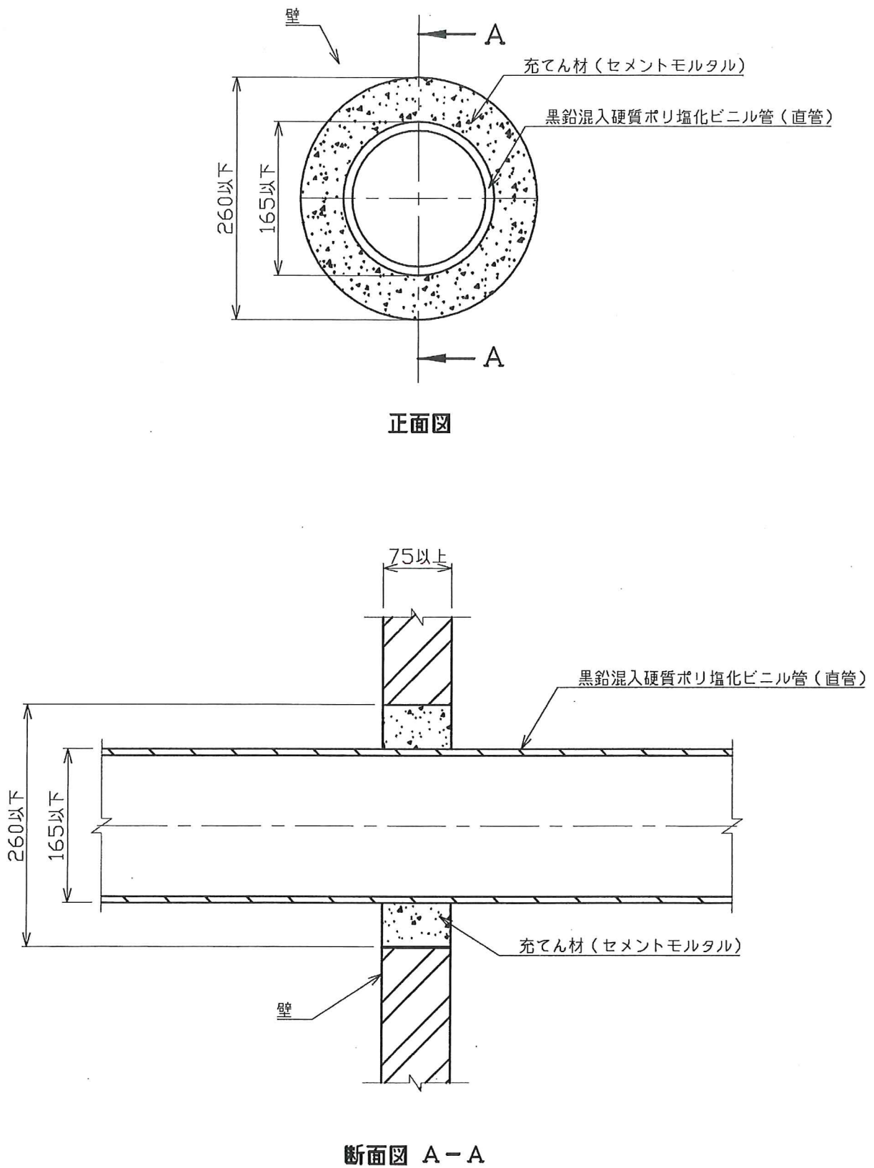
図1 構造説明図
